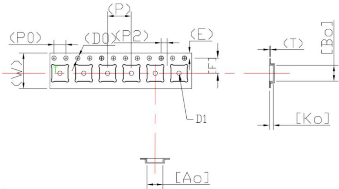
图 13：卷带尺寸图
