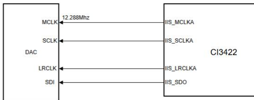
图 9: IIS 输出主模式
