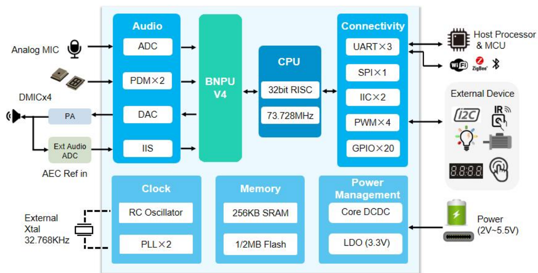
图 1：系统架构图
