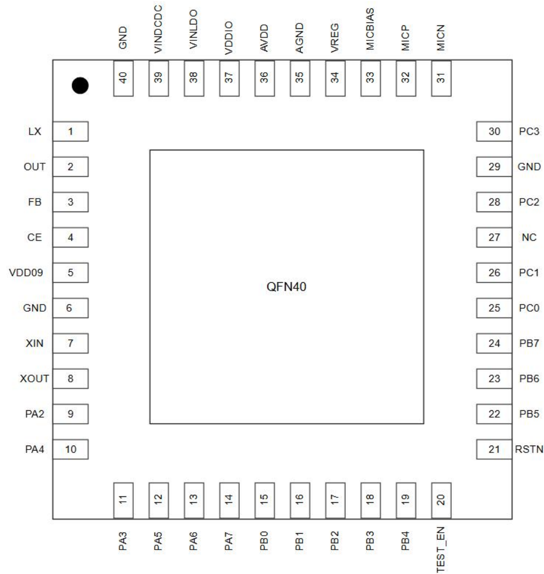
图 2：引脚图
