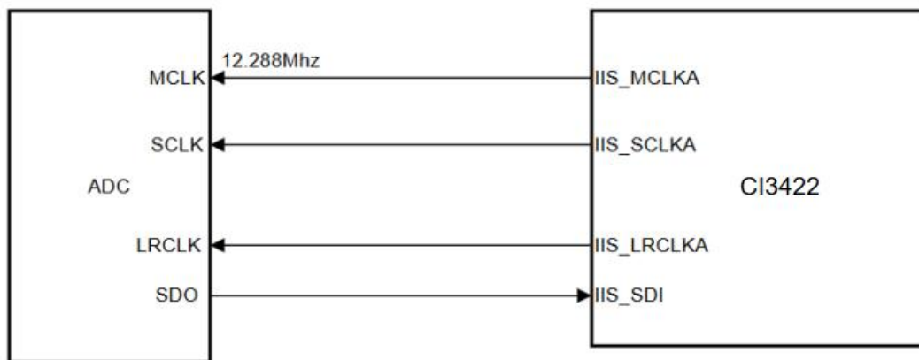
图 7: IIS 输入主模式
