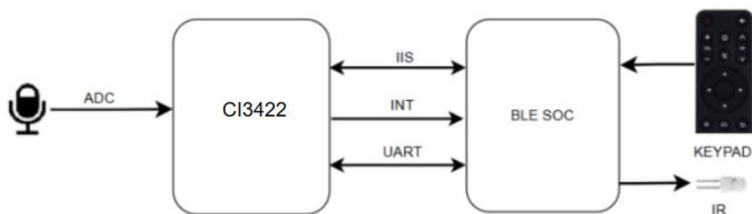
图 14： 语音遥控器应用方案示例图
