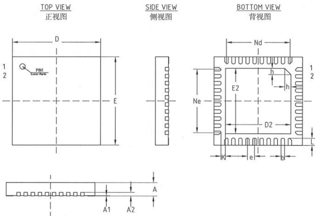
图 12: QFN40 封装尺寸
