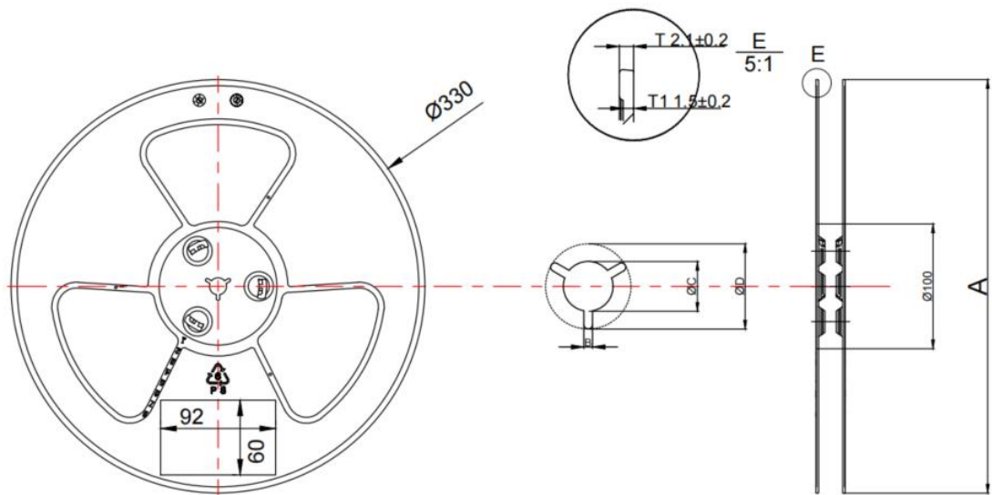
图 13：卷盘尺寸图
