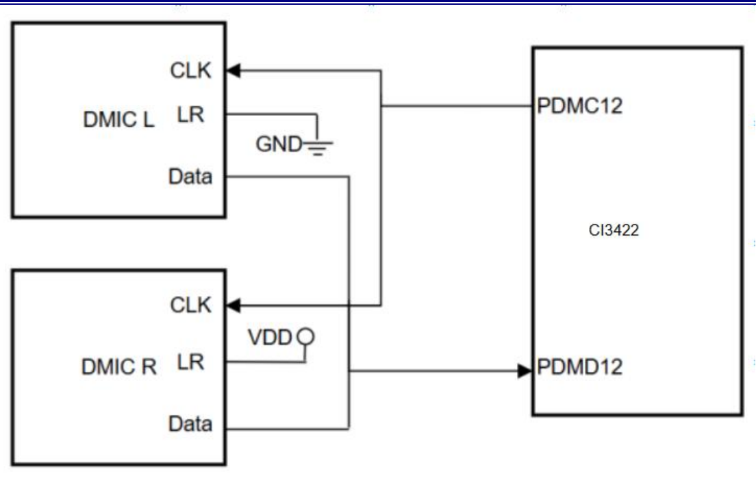
图 5: 2 路 DMIC 主模式输入
